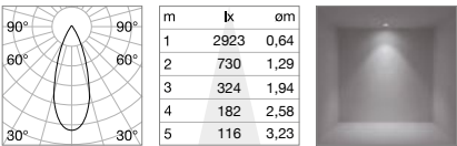
CRI≥82 15W 36° 2050lm 3000K
