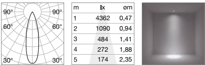
CRI≥82 15W 24° 2050lm 3000K
