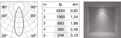
CRI≥82 30W 36° 4000lm 3000K
