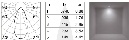
CRI≥82 30W 50° 4000lm 3000K
