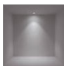
CRI ≥82 20W 36° 3000lm 3000K
