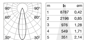
CRI ≥82 20W 24° 3000lm 3000K
