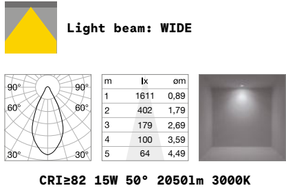
CRI ≥82 15W 50° 2050lm 3000K
