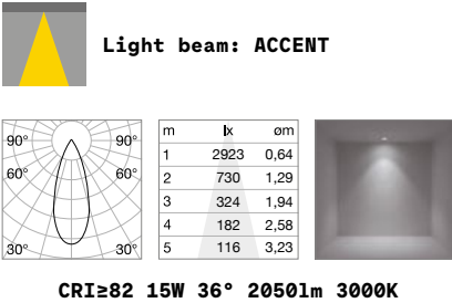
CRI ≥82 15W 36° 2050lm 3000K
