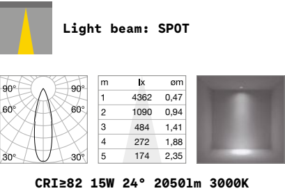
CRI ≥82 15W 24° 2050lm 3000K
