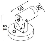
1 ■ O025FL-01B 💡 1× GU10 20 W IP 65 2 ■ O025WL-01B 💡 1× GU10 50 W IP 65
