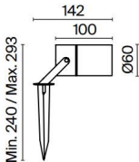
1 ■ O025FL-01B 💡 1× GU10 20 W IP 65 2 ■ O025WL-01B 💡 1× GU10 50 W IP 65
